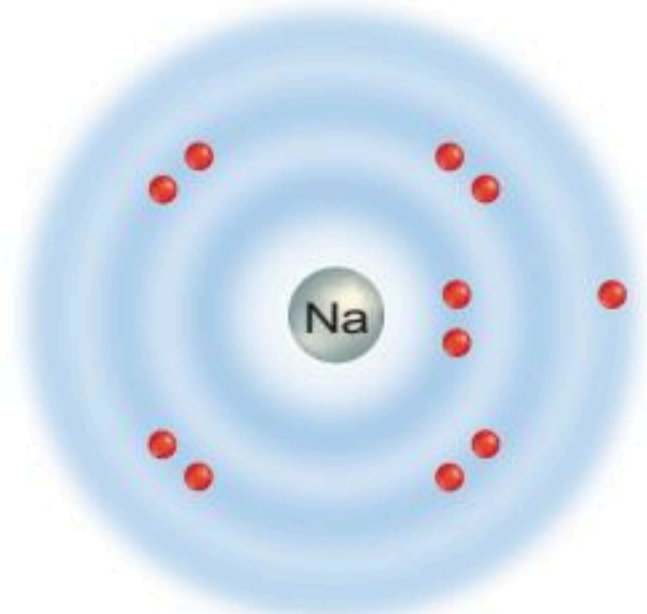
ذرة صوديوم
