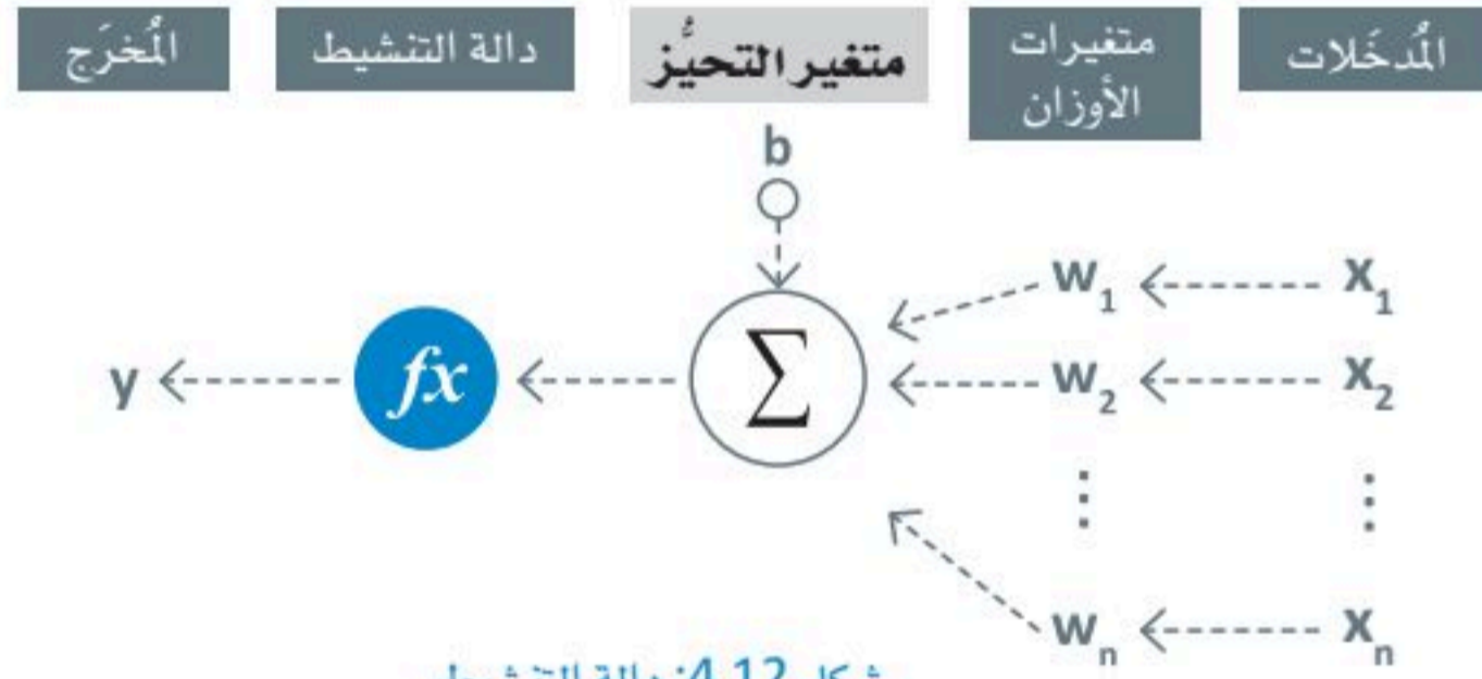
شكل 4.12: دالة التنشيط
