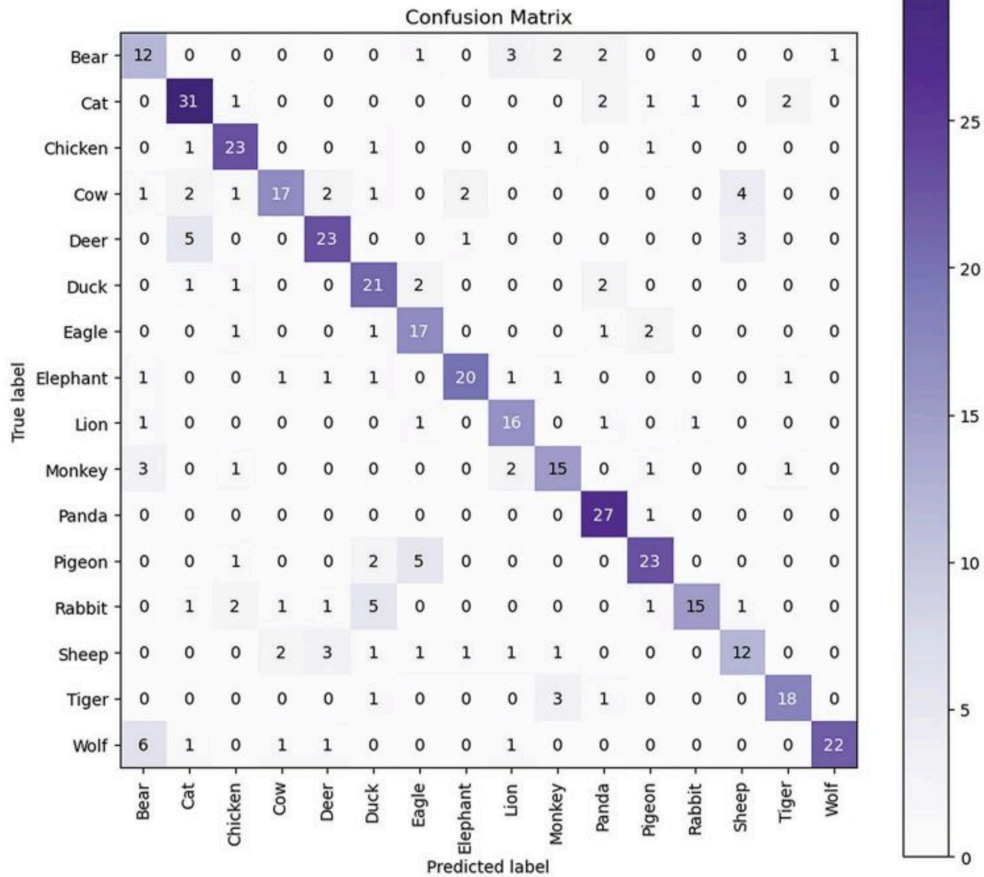
شكل 4.11: مصفوفة الدقة لأداء خوارزمية SGDClassifier
