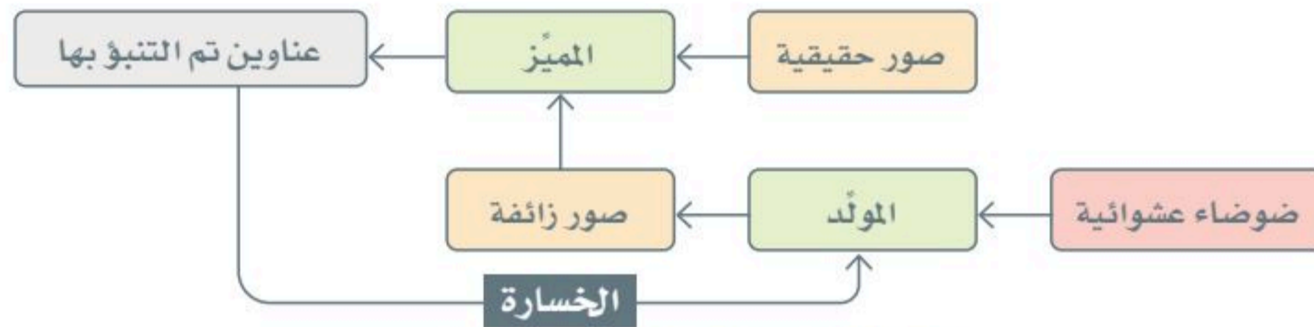
شكل 4.28: معمارية الشبكة التوليدية التنافسية
